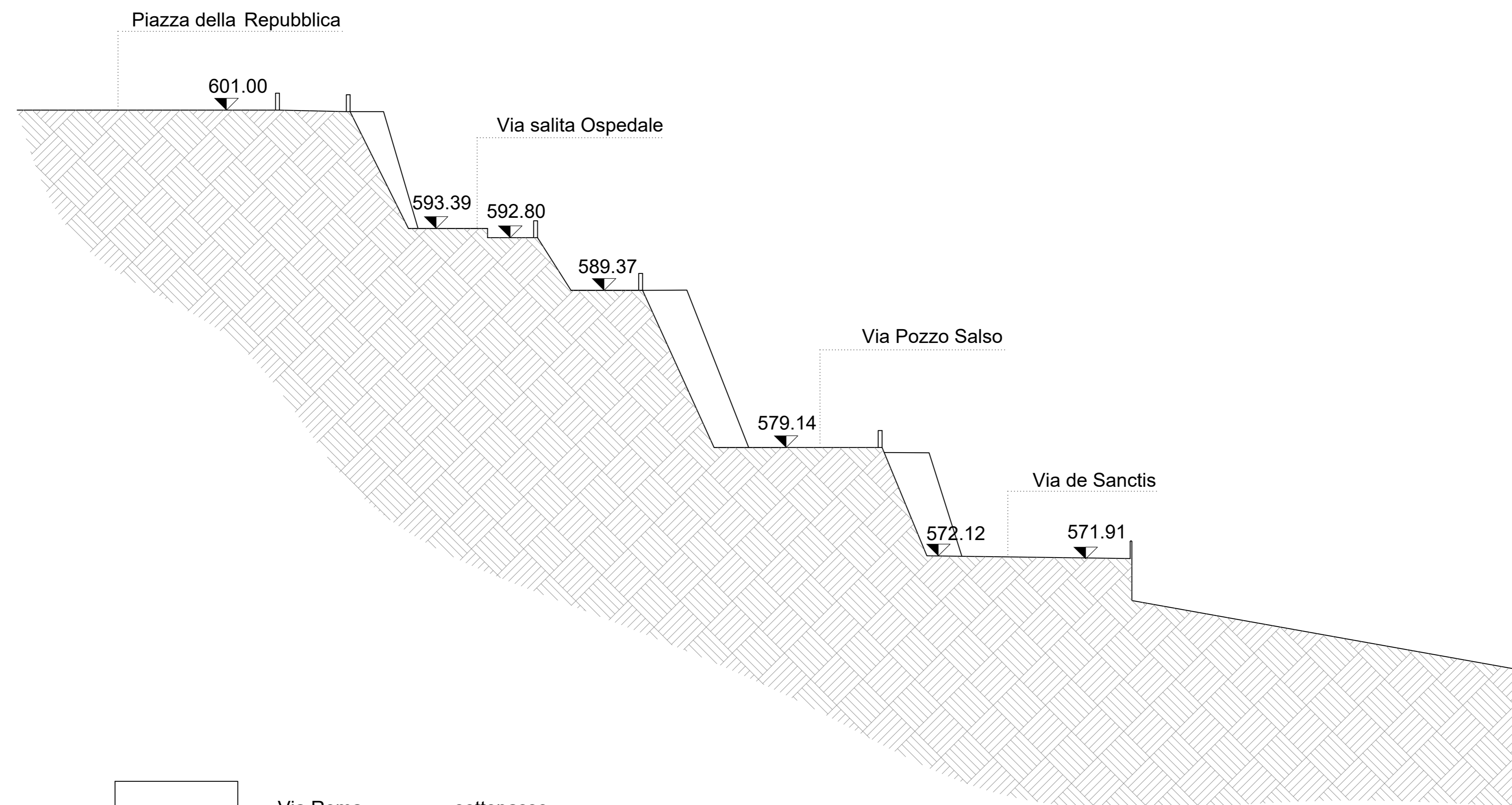
SEZIONE A-A
